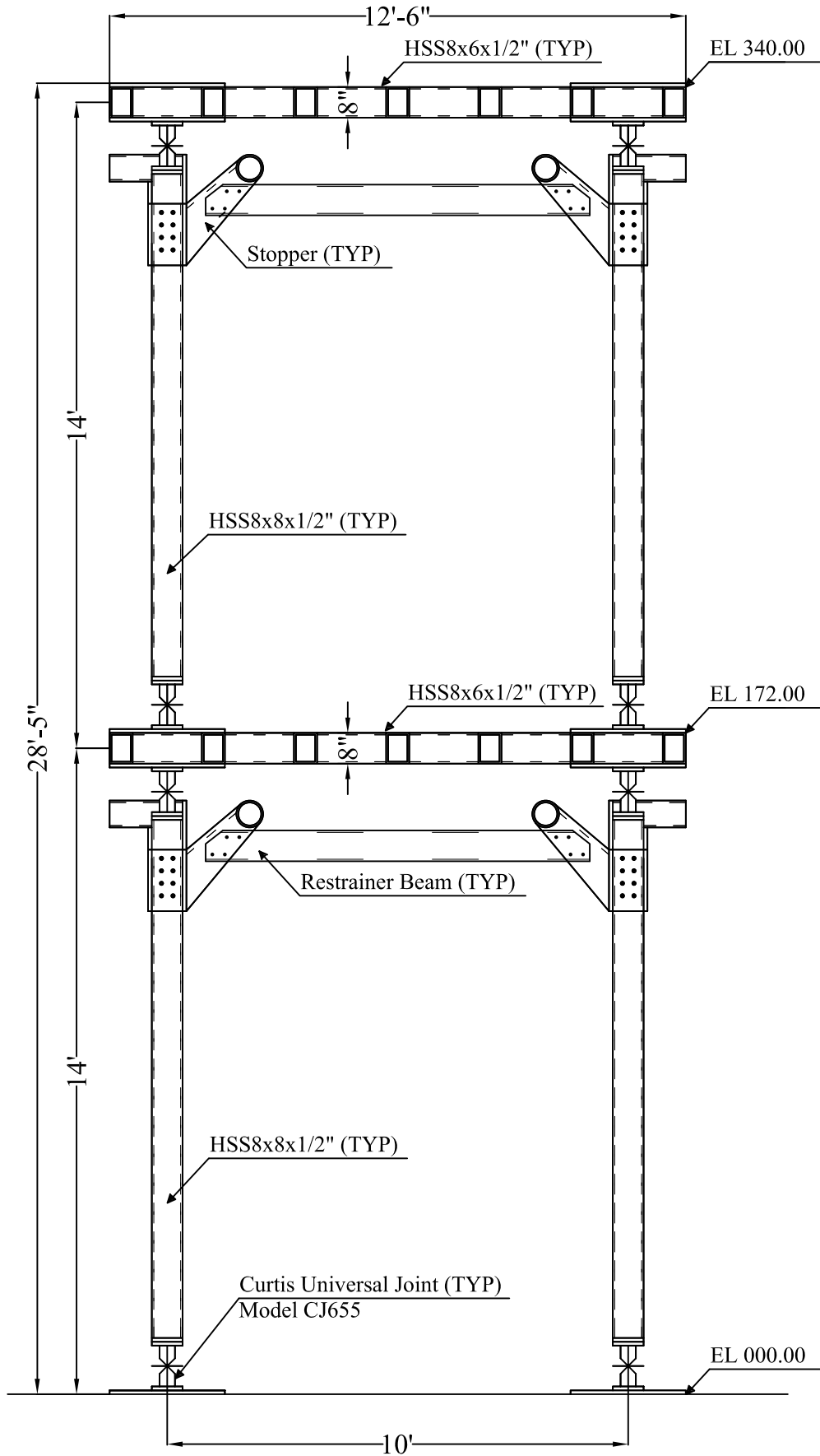
Elevation Frame
